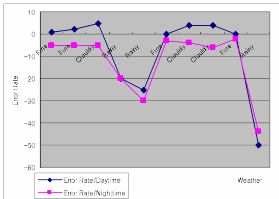
Fig. 8. Error Rate
